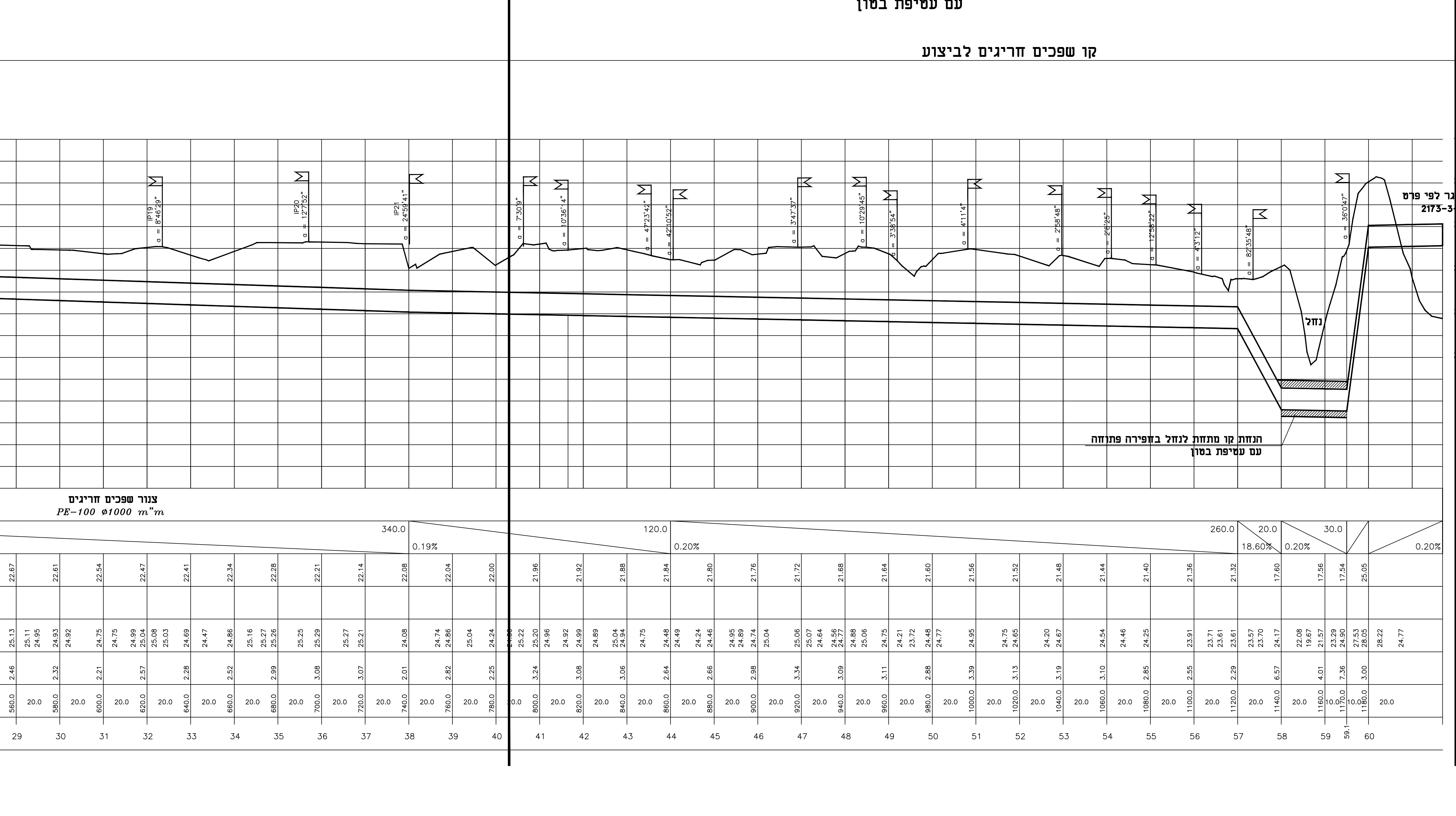
קו שפכים חריגים לביצוע עם עטיפת בטון
