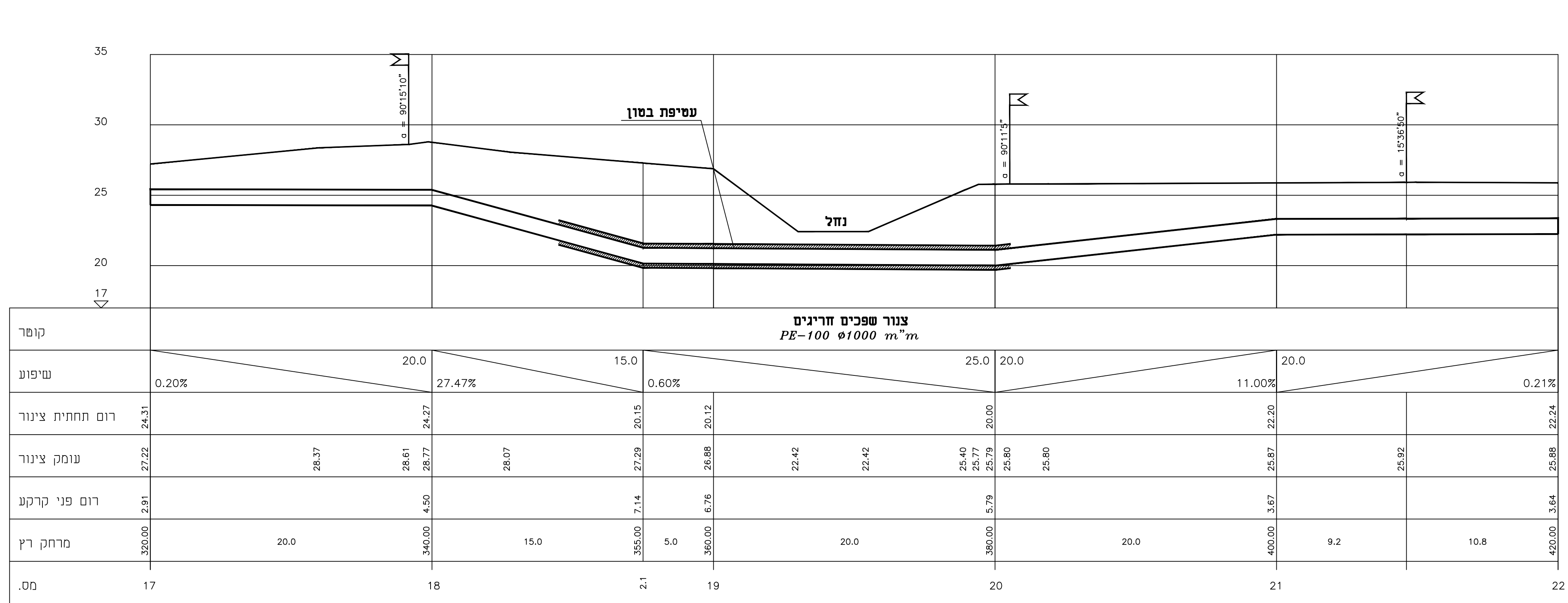
פרט 1- הנחת קו מתחת לנחל בחפירה פתוחה עם עטיפת בטון 1:200/1:200
