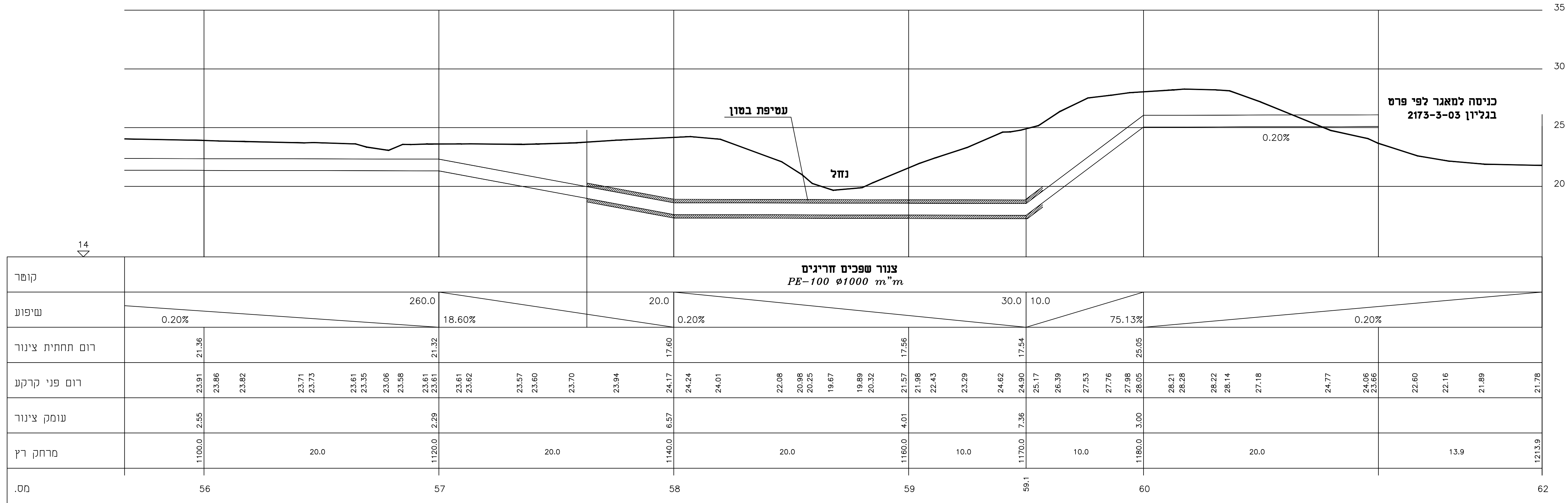
פרט 2- הנחת קו מתחת לנחל בחפירה פתוחה עם עטיפת בטון 1:200/1:200
