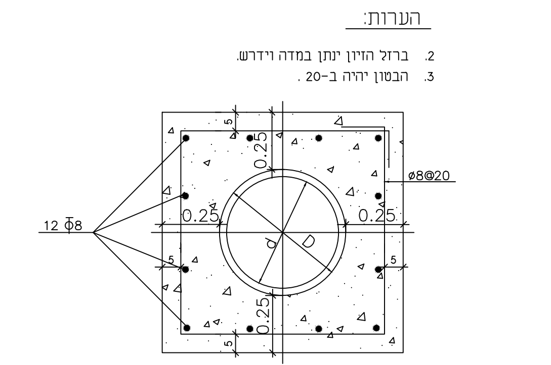
עטיפת בטון לציוור ללא קני"ח
