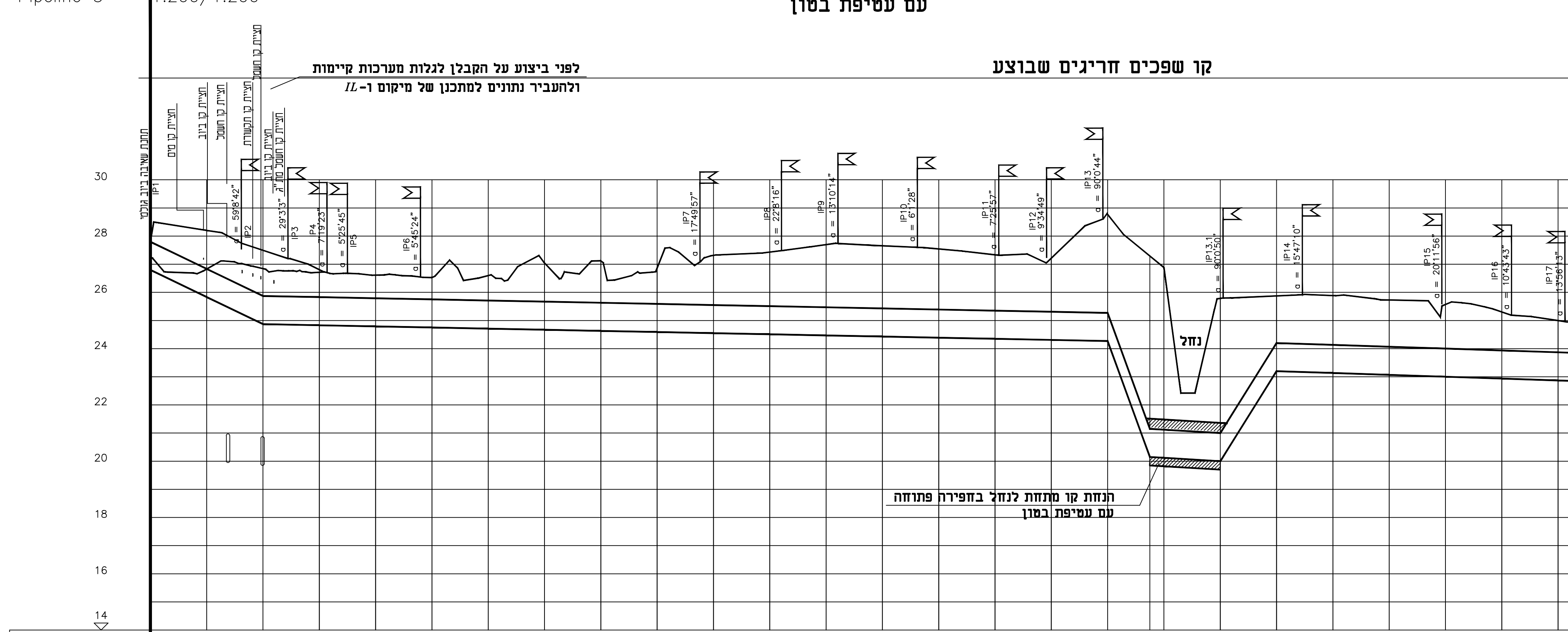
קו שפכים חריגים שבוצע לפי ביצוע על הקבלן לנחל פתוחה עם עטיפת בטון 1:100/1:1000
