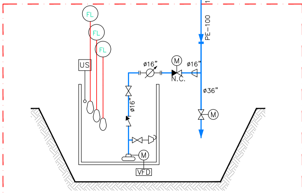
מאגר חידום שפכים חריגים תחנת שאיבה להחזרת שפכים למס"ש
