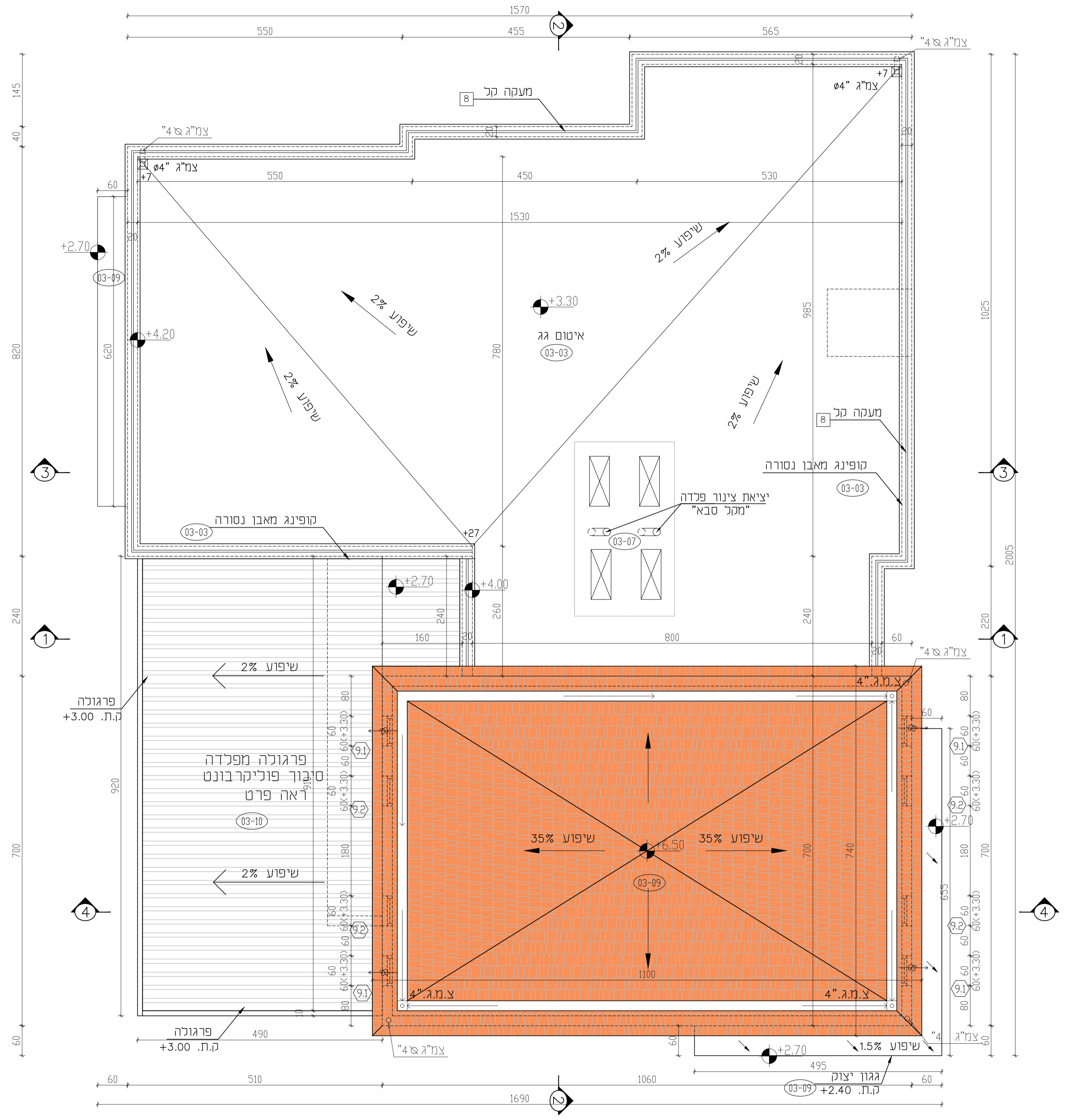
תכנית גגות
