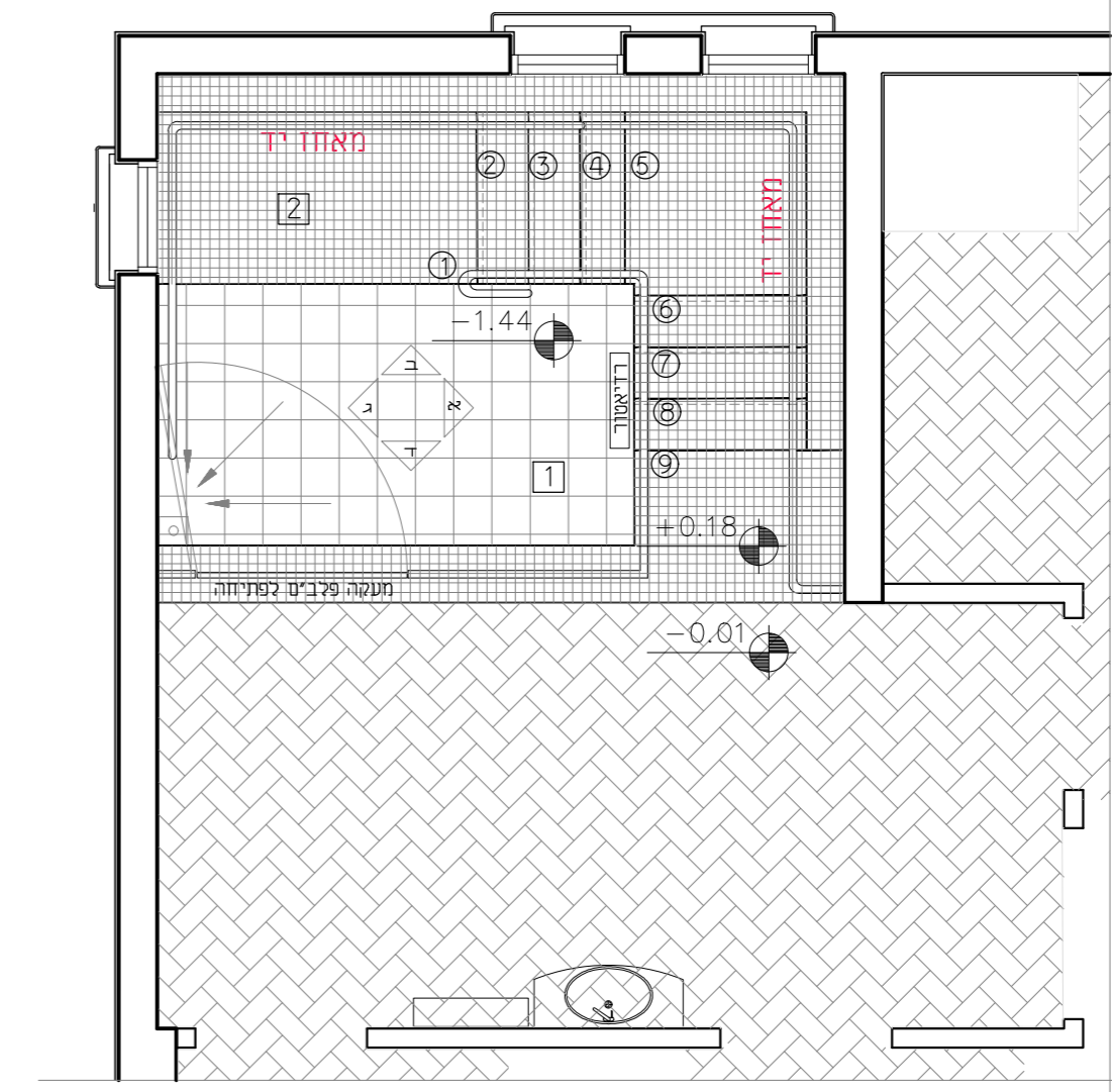
חדר טבילה-תכנית
