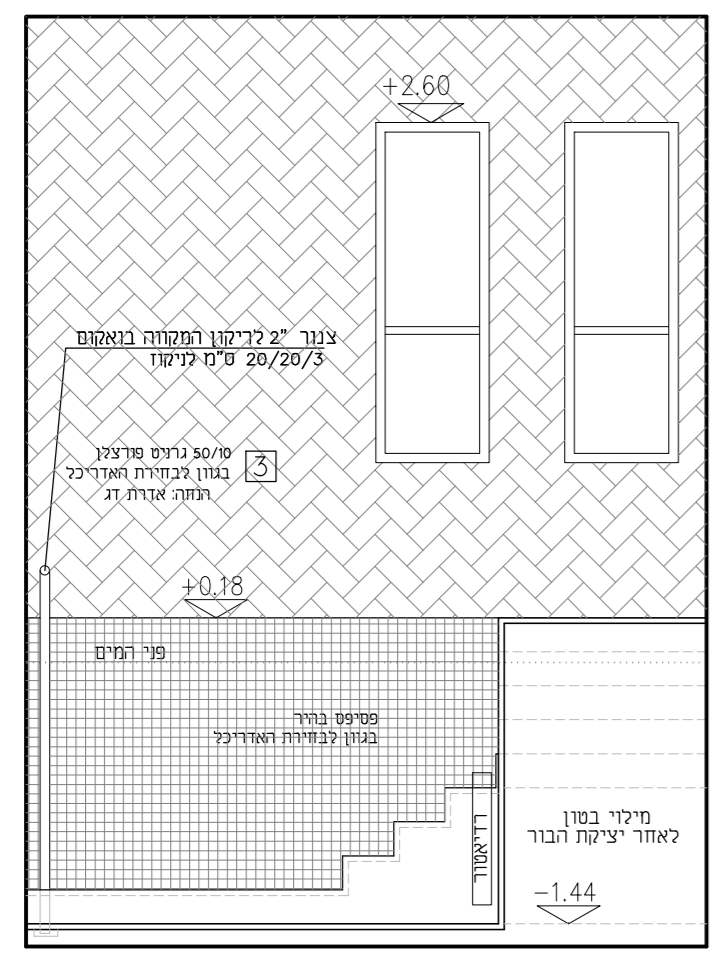
מבט ב
